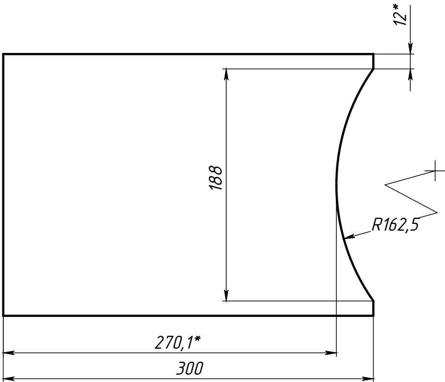
Поз.1 (Основание)
